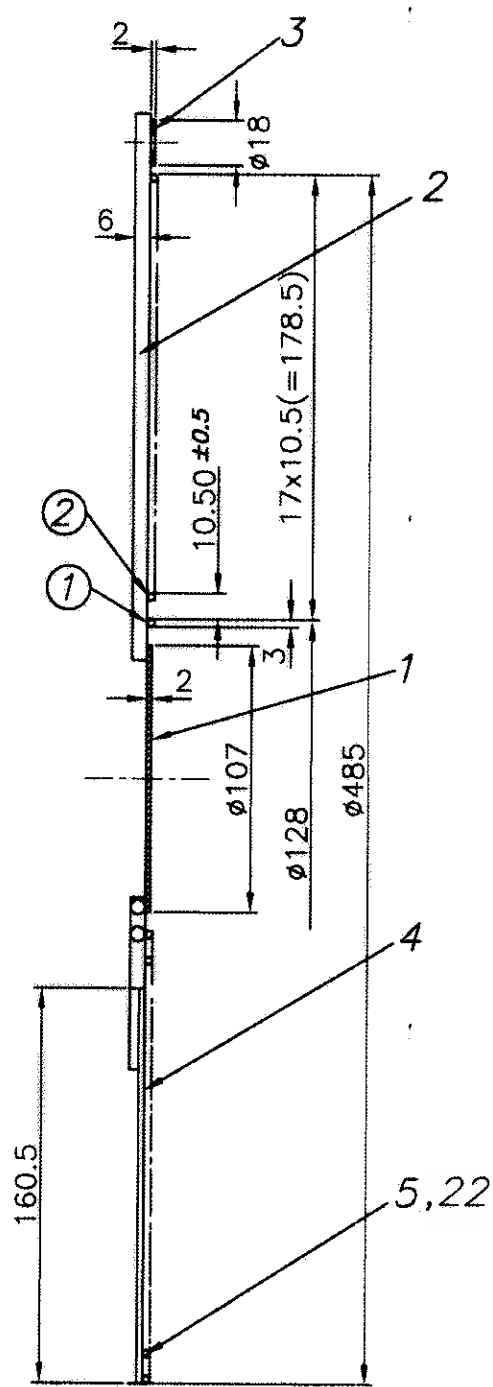
SECTION A-A
